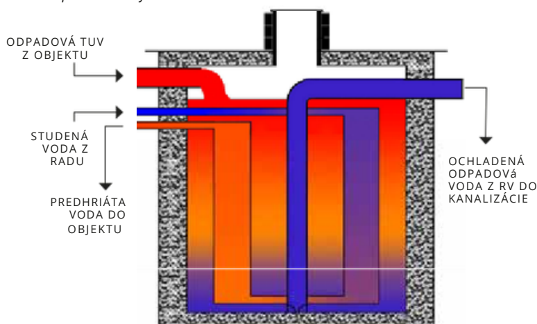
Schéma rozloženia teplôt v rekuperačnom výmenníku
