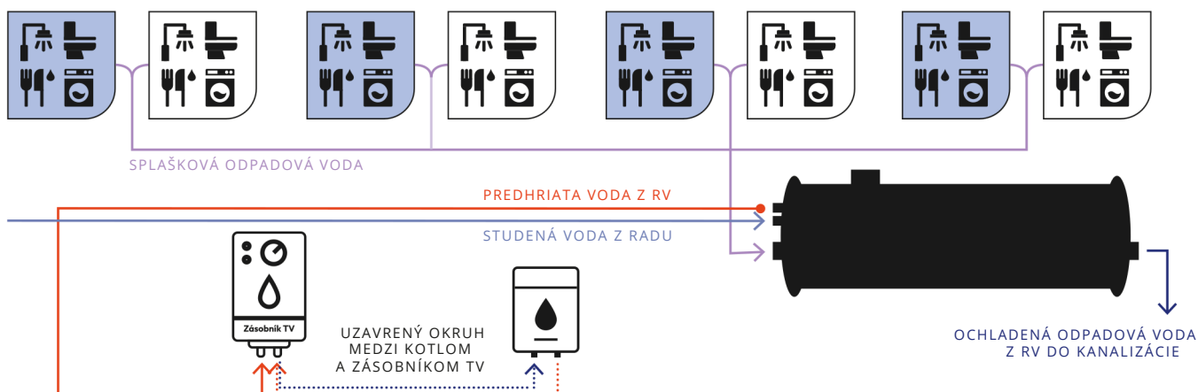
Schéma zapojenia rekuperačného výmenníku (RV) v bytovom dome
